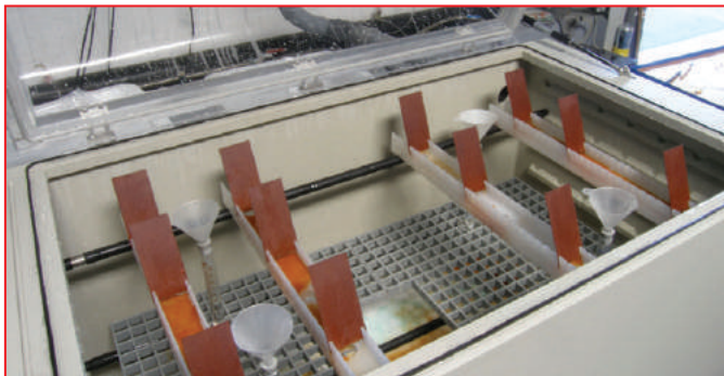
Câmara para teste de corrosão do aço inoxidável em nevoeiro salino. Chamber for STAINLESS STEEL corrosion tests in a saline mist.
