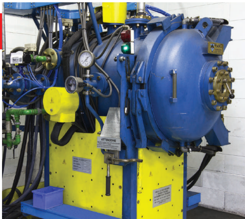
Forno de têmpera a vácuo para tratamento térmico. Vacuum furnace for heat treatment.
